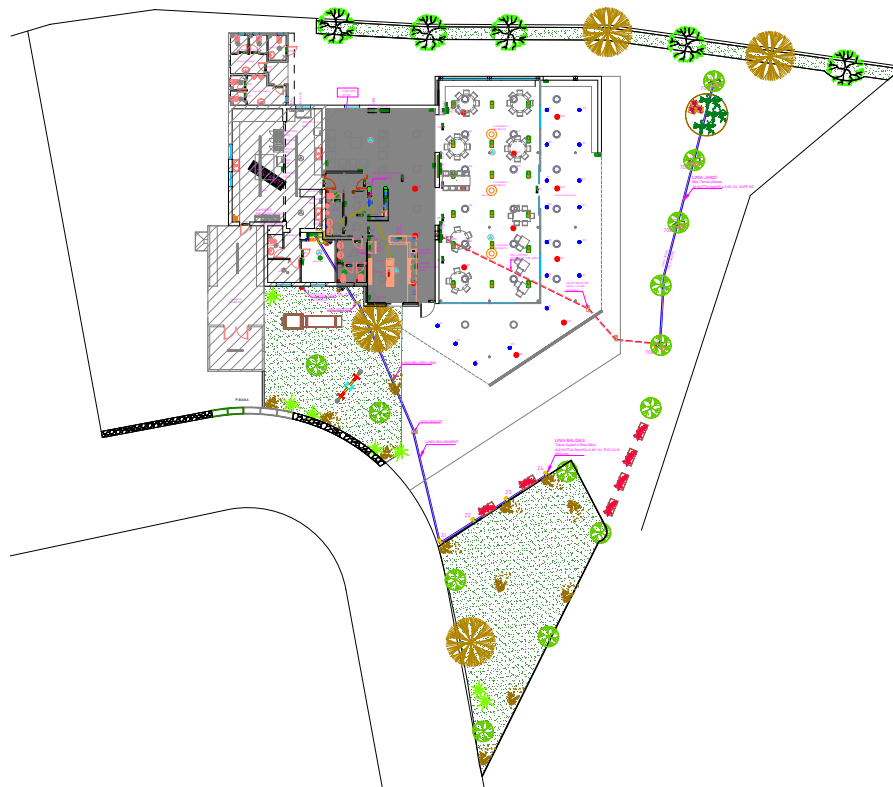
PLÀNOL INSTAL·LACIONS
